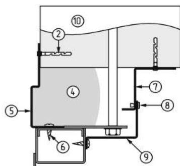
Пример монтажа наличников Вид сбоку
