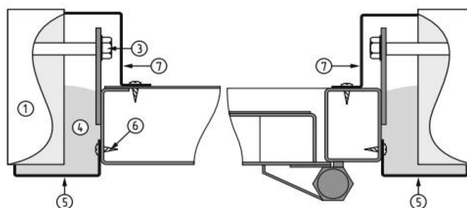
Пример монтажа наличников Вид сверху
