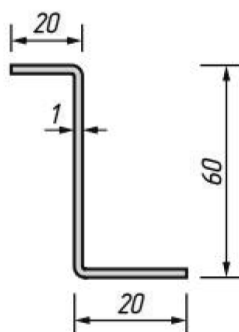
КНВЛ-20-210(250)
